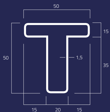
16B Kg/m 2,33
