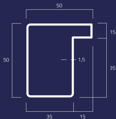
16A Kg/m 2,33
