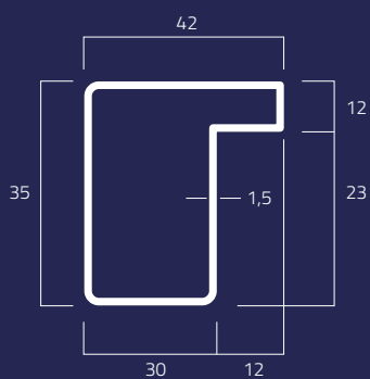
2A Kg/m 1,76
