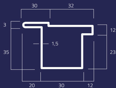
2T Kg/m 2,30
