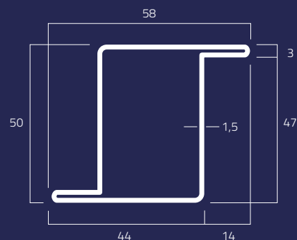
SF3B Kg/m 2,52
