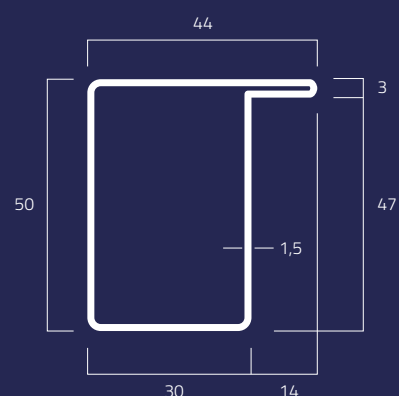
SF1B Kg/m 2,15
