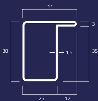
1A Kg/m 1,72
