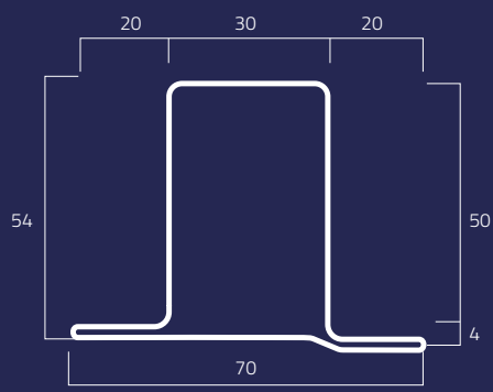
F26B
