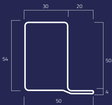
F26A
