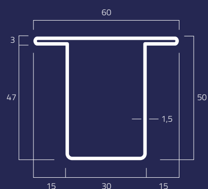
SF2B Kg/m 2,52
