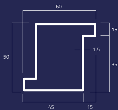
16Z Kg/m 2,56
