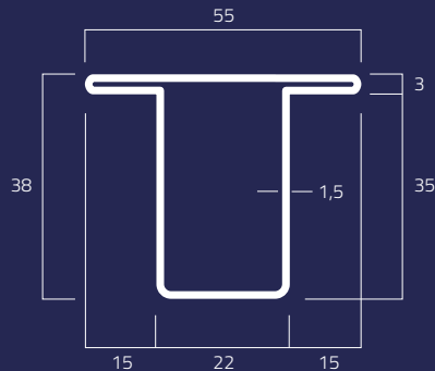
1B Kg/m 2,10
