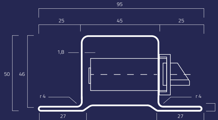
TS20T Kg/m 4,00
