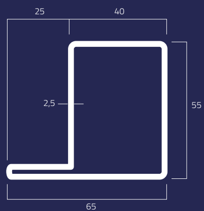
T770 Kg/m 4,53
