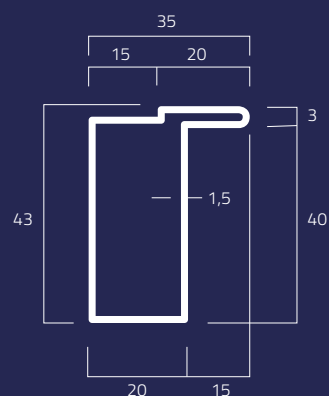
14A Kg/m 1,79
