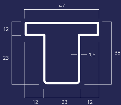
2B Kg/m 1,88
