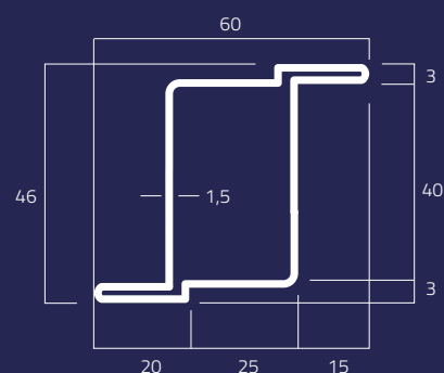
15Z Kg/m 2,45
