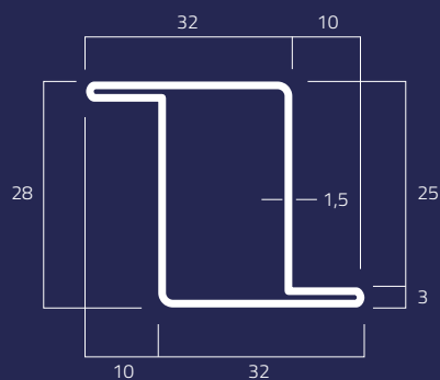
11C Kg/m 1,57
