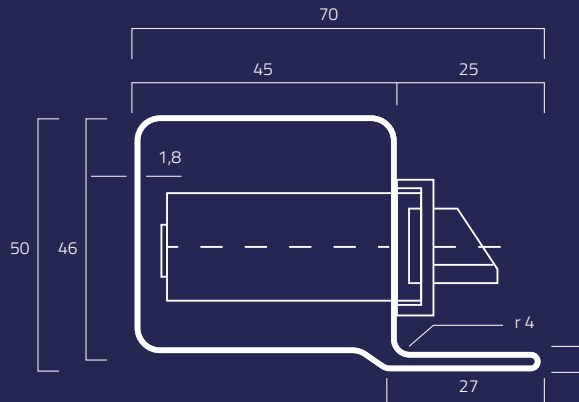
TS20L Kg/m 3,33
