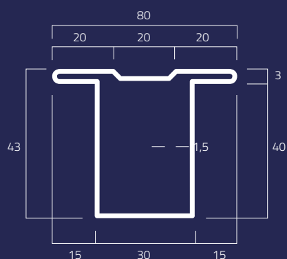
15T Kg/m 2,45
