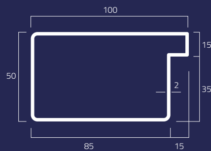
16D Kg/m 4,65
