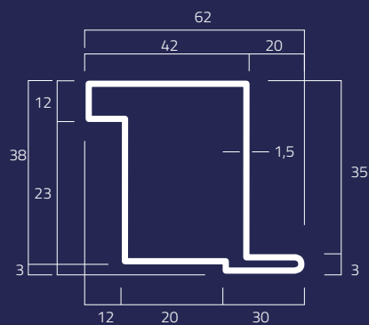
2N Kg/m 2,30
