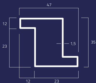
2Z Kg/m 1,88
