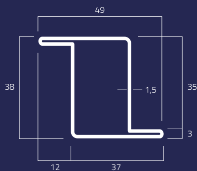
1C Kg/m 1,99
