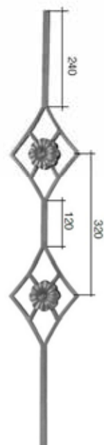
Art. 303A04 \Phi 14 mm H.1000 mm L.160 mm
