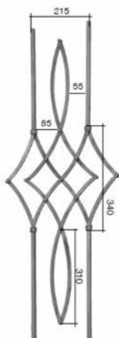
Art. 302B05 \phi 12 mm H.1000 mm L. 415 mm
