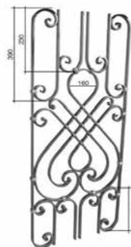
Art. 311A07 ∅16 x 8 mm H.1000 mm L.420 mm
