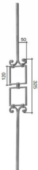
Art. 302A04 \phi 14 mm H.1000 mm L.115 mm
