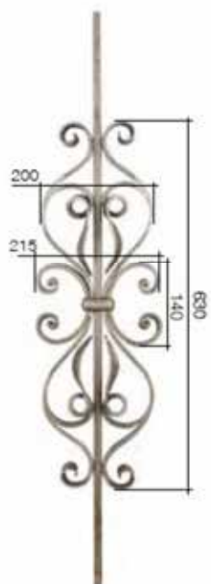
Art. 304A04 φ 14 mm H.1000 mm L. 215 mm
