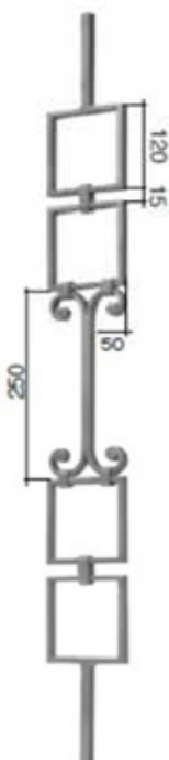
Art. 302A05 \phi 14 mm H.1000 mm L.115 mm
