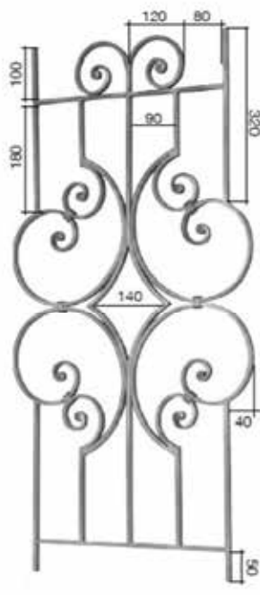
Art. 312A07 ∅14 x 8 mm H. 1000 mm L. 500 mm
