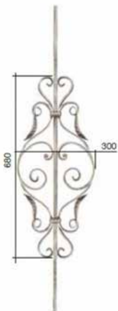
Art. 304A01 φ 14 mm H.1000 mm L. 300 mm
