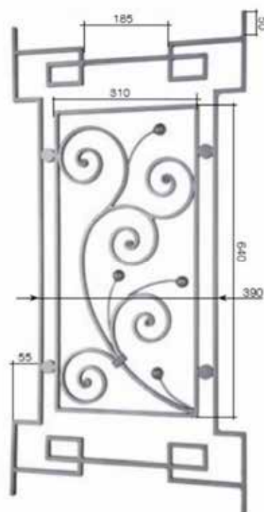
Art. 310A05 ∅14X8mm H.1000 mm L.500 mm
