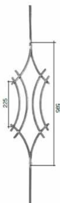
Art. 302B06 \phi 12 mm H.1000 mm L. 200 mm
