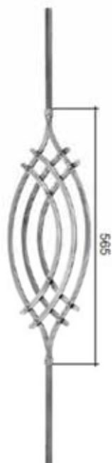
Art. 302B02 \phi 12 mm H.1000 mm L. 200 mm
