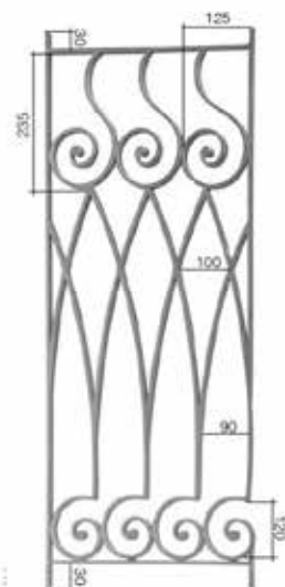
Art. 311A03 ∅14 x 8 mm H.1000 mm L. 395 mm
