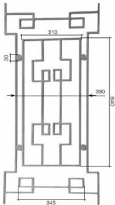
Art. 310A01 ∅14X8mm H.1000 mm L.500 mm
