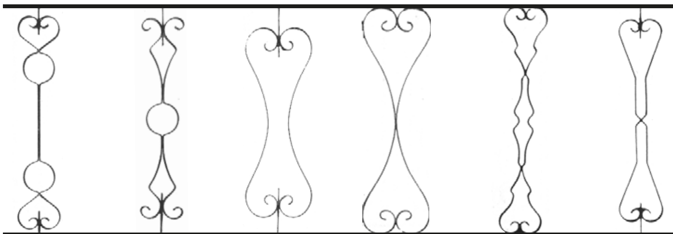
49A01 □ 20x4 49A04 □ 20x4 49A07 □ 20x4 49A10 □ 20x4 49A13 □ 20x4 49A16 □ 20x4 49A02 □ 25x4 49A05 □ 25x4 49A08 □ 25x4 49A11 □ 25x4 49A14 □ 25x4 49A17 □ 25x4 49A03 □ 30x4 49A06 □ 30x4 49A09 □ 30x4 49A12 □ 30x4 49A15 □ 30x4 49A18 □ 30x4 H 800 mm H 800 mm H 800 mm H 800 mm H 800 mm H 800 mm
