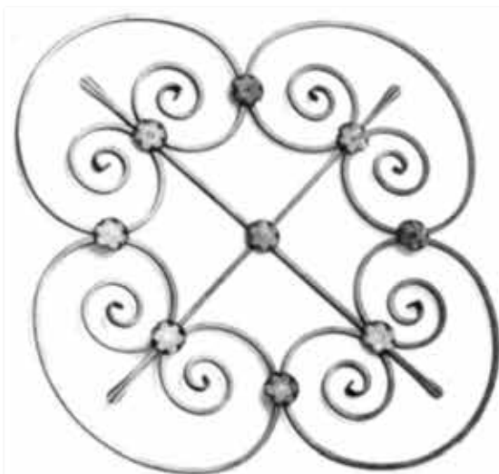
Art. 8A02 Ø 810 mm φ 10 mm
